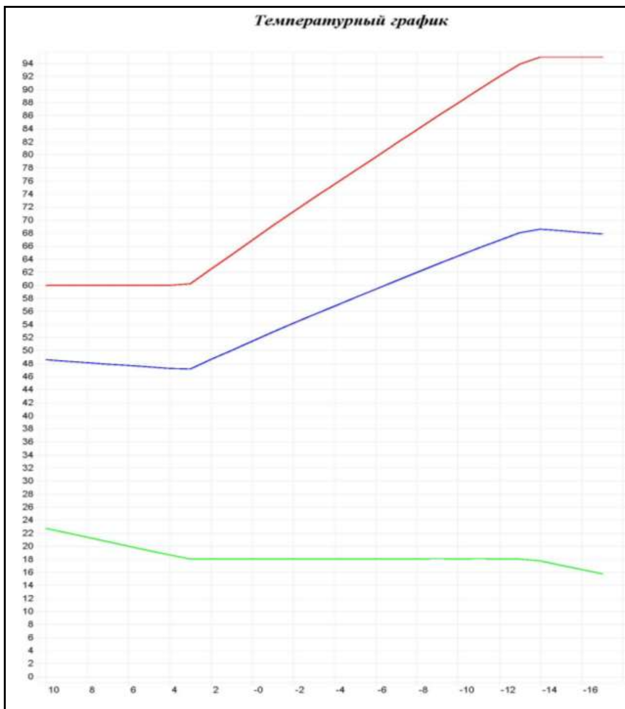
Рисунок 5.8.1 – Расчет отпуска тепловой энергии для котельной Батуринского сельского поселения Брюховецкого района в течение года при температурном графике 95-70 °С
