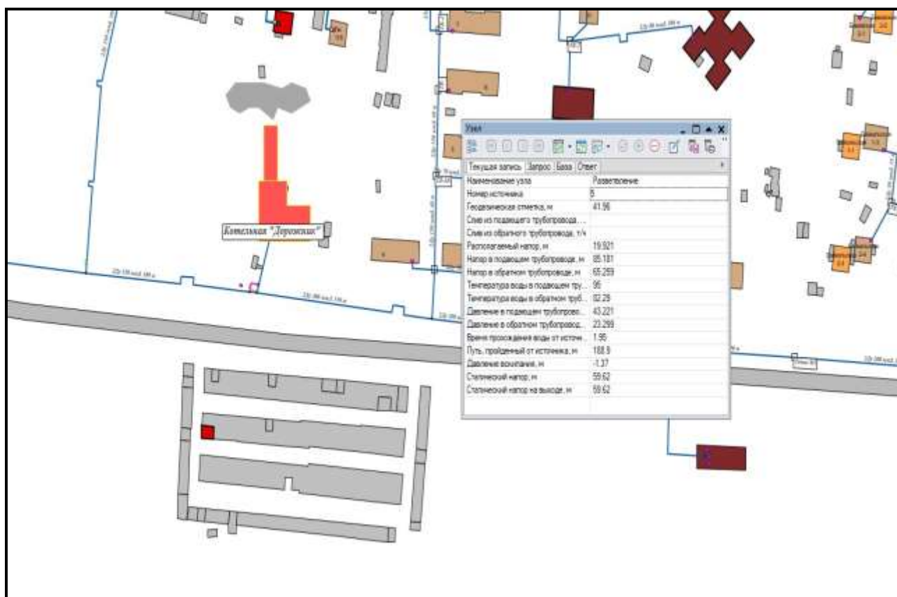
Рисунок 3.2.3 – Паспорт объекта теплоснабжения «Узел»
