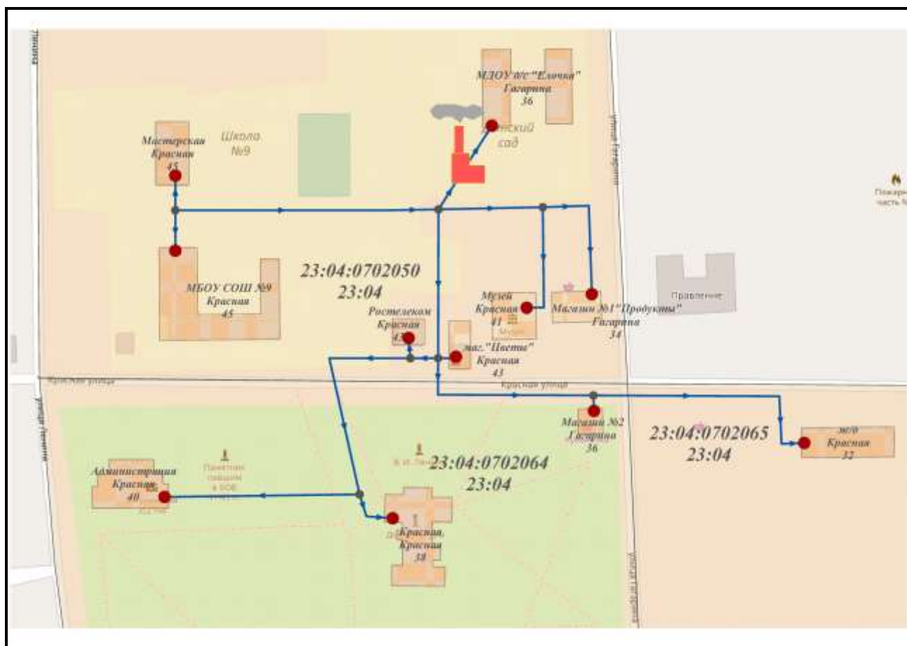
Рисунок 2.4.1 – Зона действия ВОК (кадастровый квартал)
