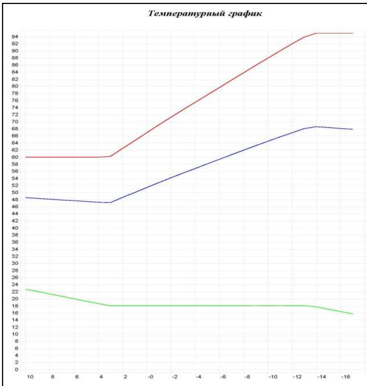
Рисунок 1.2.7.1 – График изменения температур теплоносителя 95–70 °С
