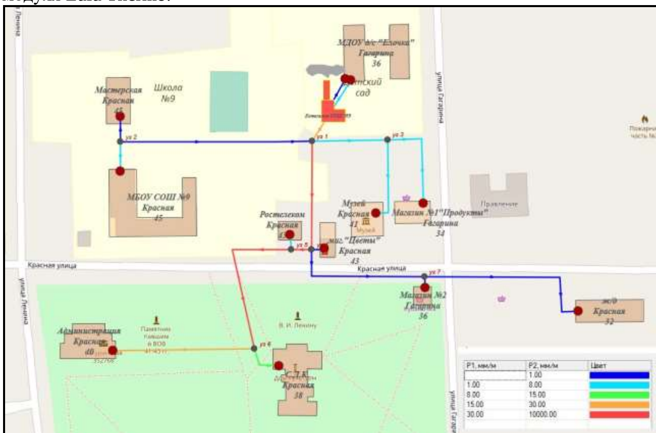
Рисунок 4.2.1 – Пропускная способность теплосетей (в цвете)
