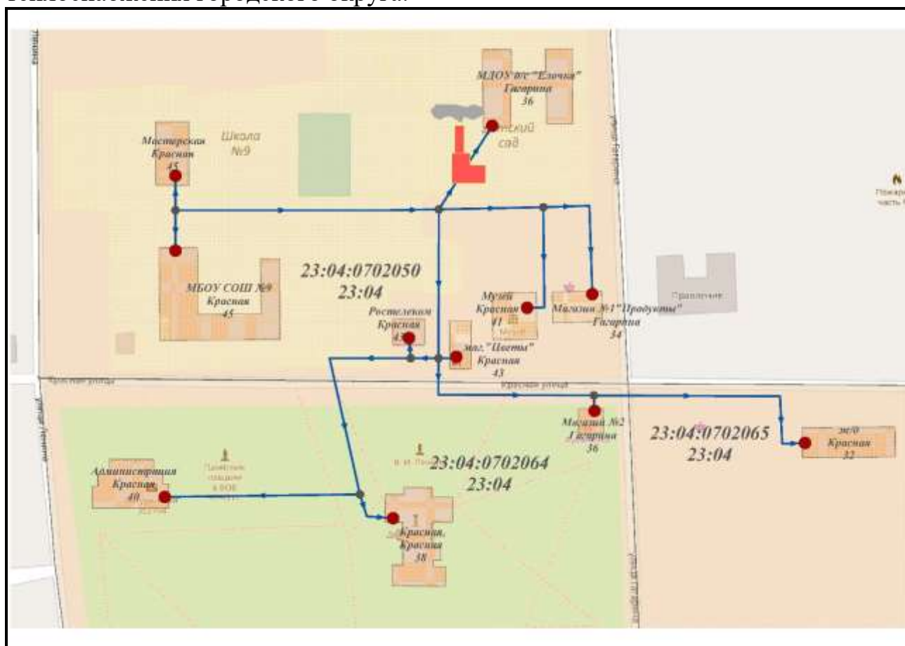
Рисунок 3.3.1 – Отражение кадастровых кварталов на схеме теплоснабжения
