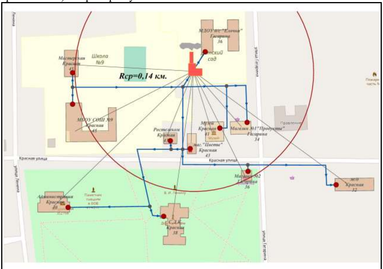
Рисунок 2.5.1 – РЭС ВСК
